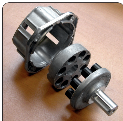
Joint élastique pour un meilleur accouplement de la pompe (modèle triphasé)
